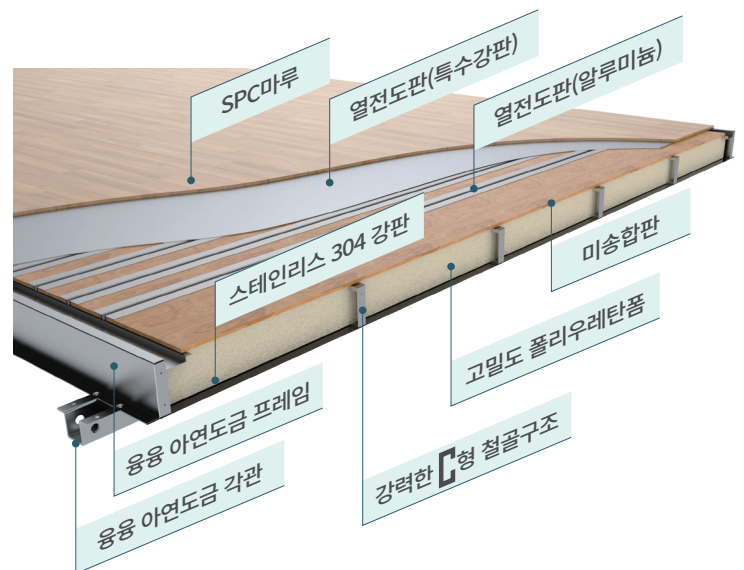
바닥온돌난방구조
